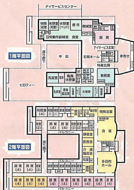
特養ゆのさと園平面図
